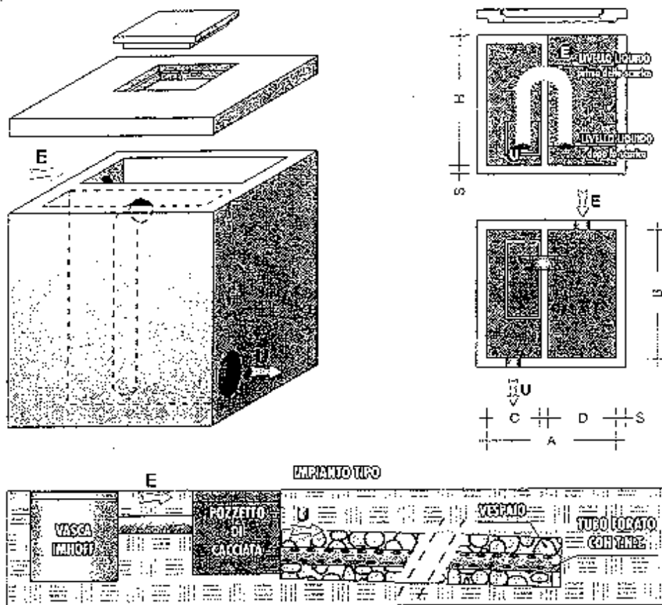
Schema 3: Esempio di pozzetto di cacciata.
